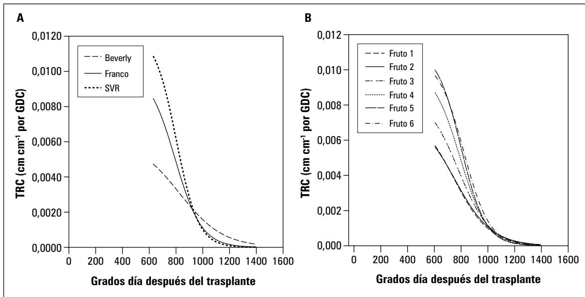
Figura 3. Comportamiento de la tasa relativa de crecimiento (TRC) del fruto de tomate en tiempo fisiológico de (A) tres híbridos y (B) afectado por la ubicación del fruto en el primer racimo.
