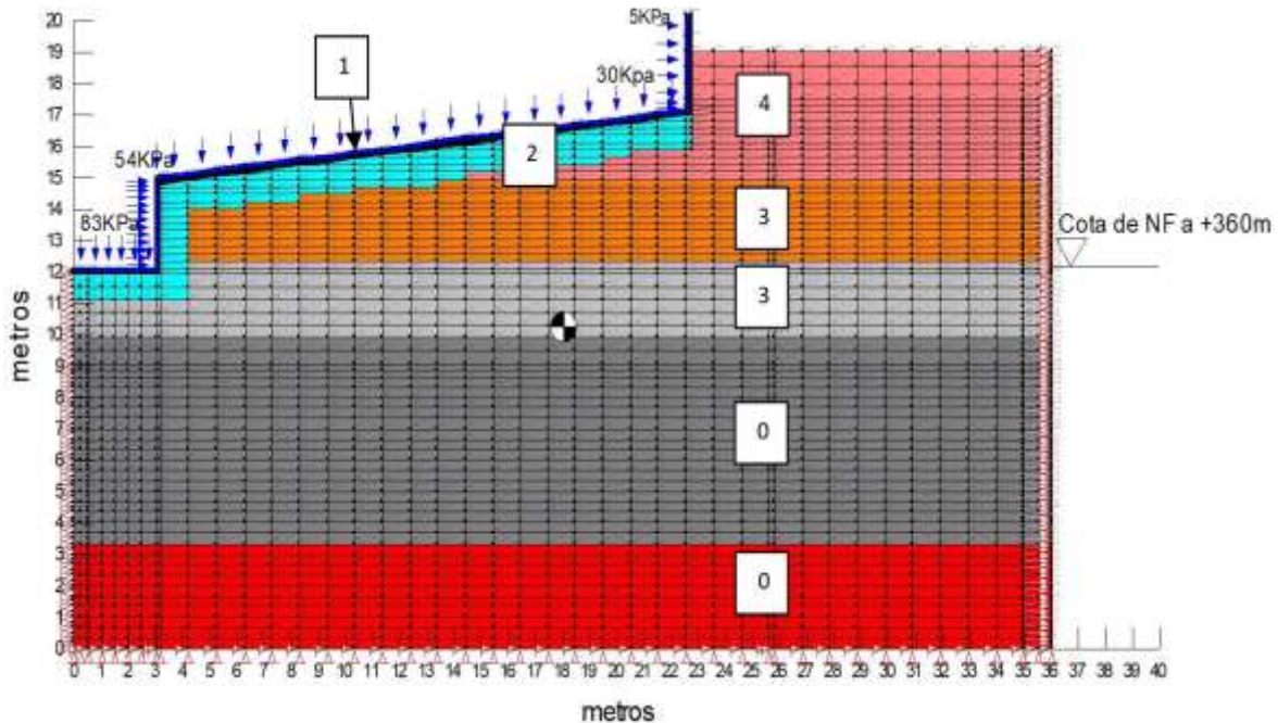
Fig. 5. Malla de elementos finitos (nudos y elementos), condiciones de apoyo, condiciones de borde, estado de carga, estratos de suelos y etapas constructivas.
