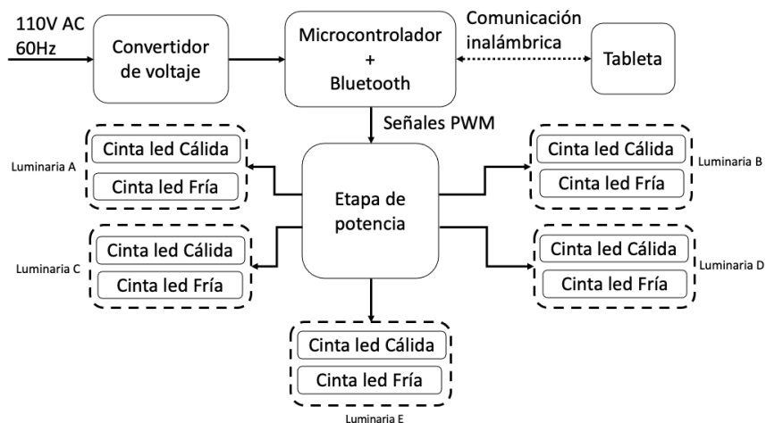
Fig. 2. Diagrama de bloques del Sistema de Iluminación Dinámica.
