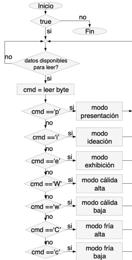
Fig. 4. Diagrama de flujo con la descripción del algoritmo que fue implementado en el sistema de iluminación dinámica.
