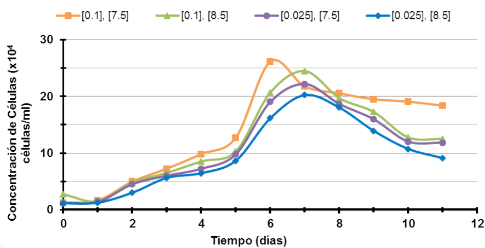
FIG. 3. Curva de crecimiento de Chlorella sp. Los números en corchetes corresponden a la concentración de nitrógeno y pH, respectivamente. El valor reportado es el promedio de las mediciones de las dos repeticiones.
