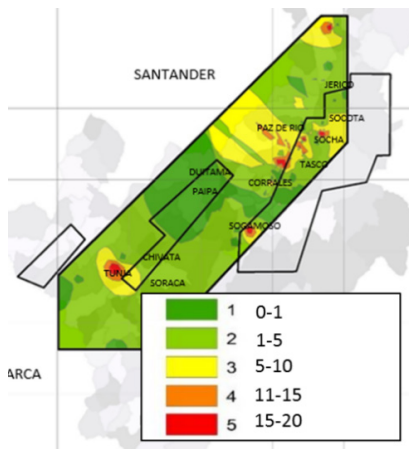
Figura 3. Mapa IDW de intervalos de contenido de gas del polígono de estudio.
