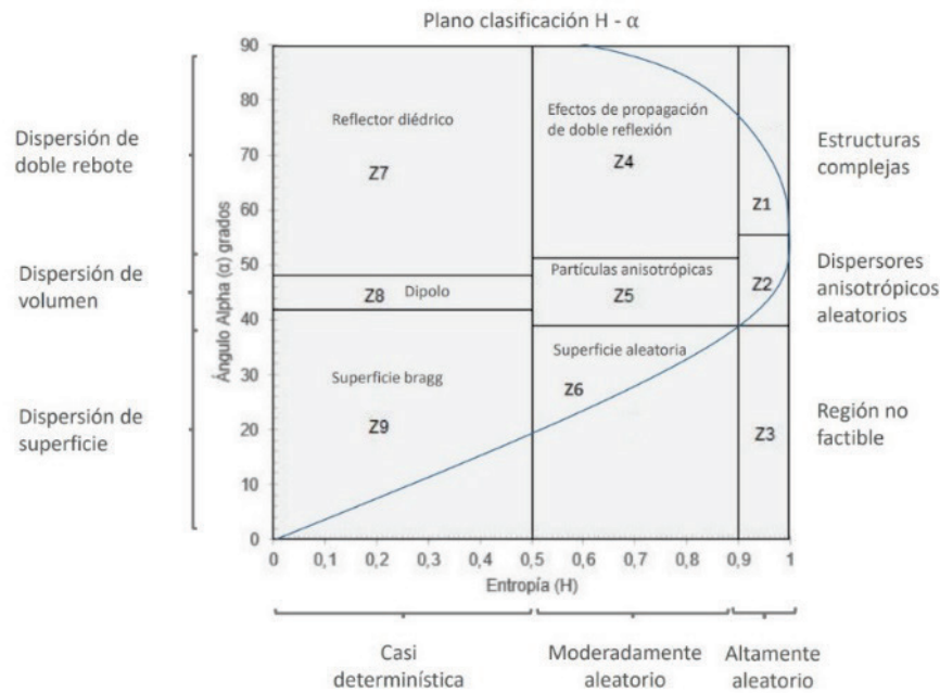
FIGURA 1. Plano de clasificación H - \alpha
